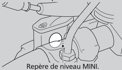
Réservoir de liquide de frein avant
