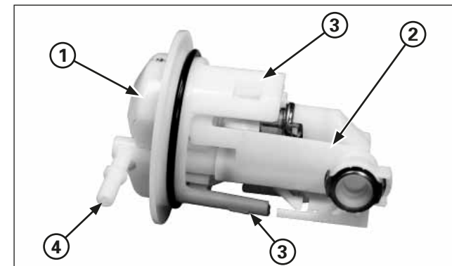
(1) POMPE (3) ÉTRIER (2) CORPS (4) TUBE DE CONNEXION
