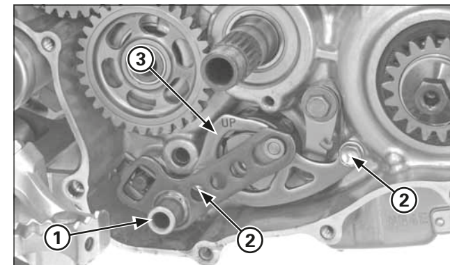
(1) AXE STRIÉ DE LA BOÎTE (2) VIS (3) PLAQUE DU GUIDE
