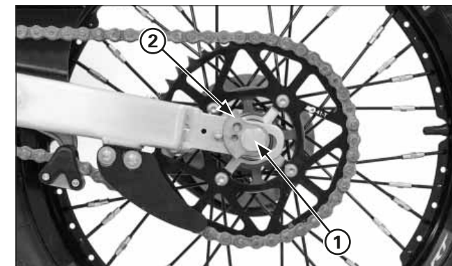
(1) AXE (2) TENDEURS
