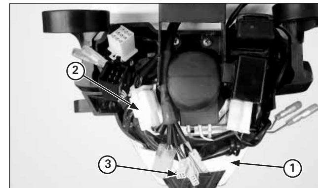
(1) BOÎTIER DU PHARE SUPÉRIEUR (2) CONNECTEUR 6P (3) CONNECTEUR 3P
