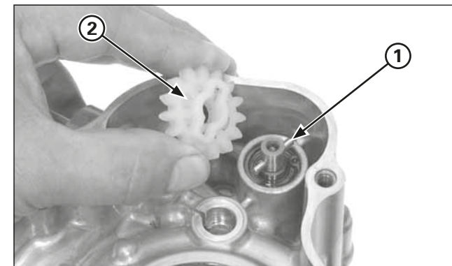
(1) ARBRE MENANT (2) COURONNE DE TRANSMISSION SECONDAIRE
