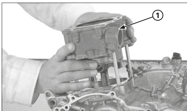
(1) CYLINDRE
